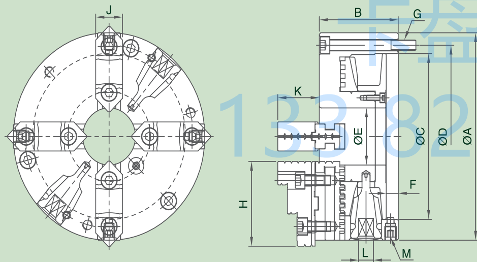
尺寸圖 » Dimensions
